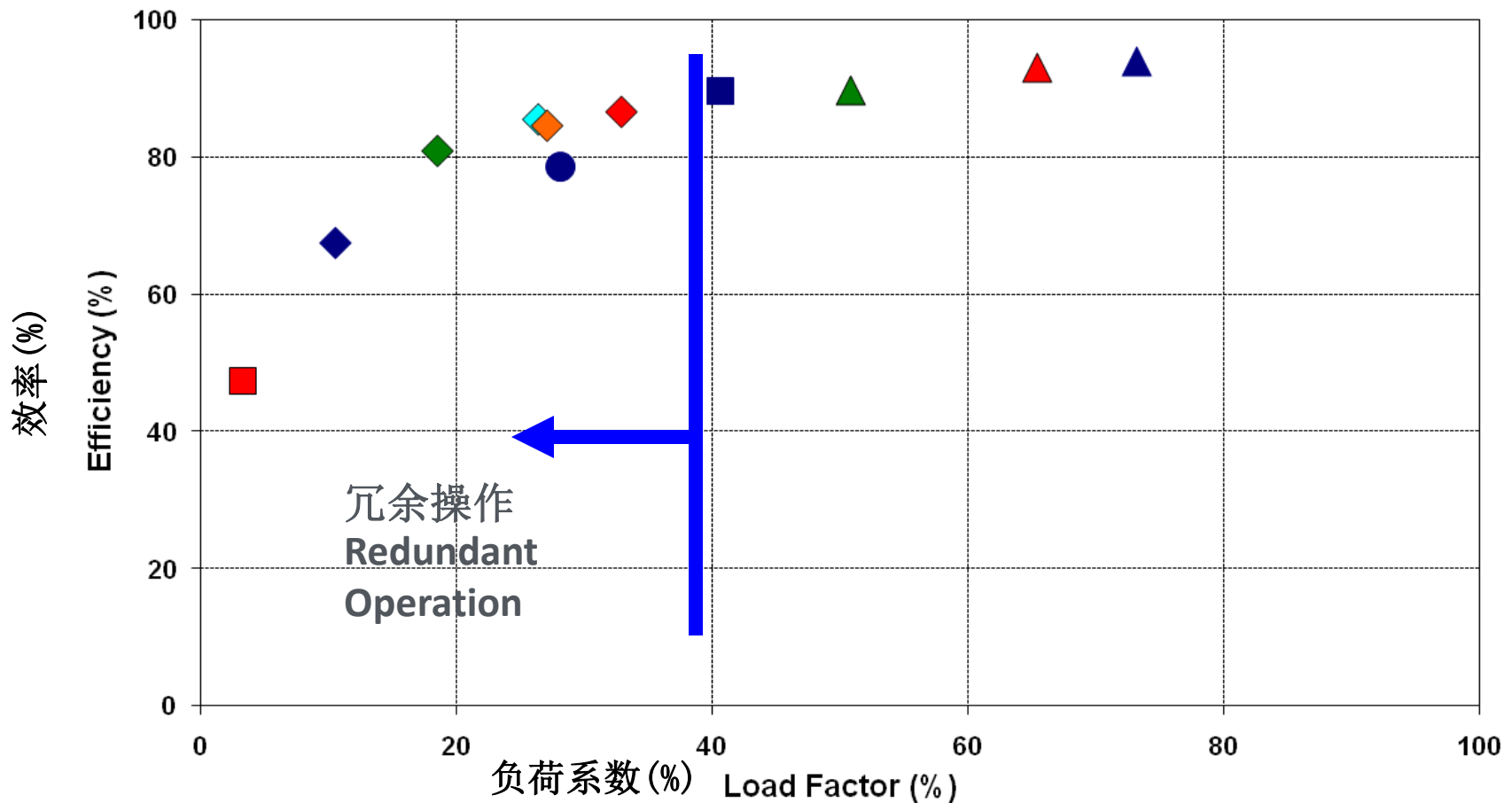
不间断电源系统的效率 UPS Efficiency
