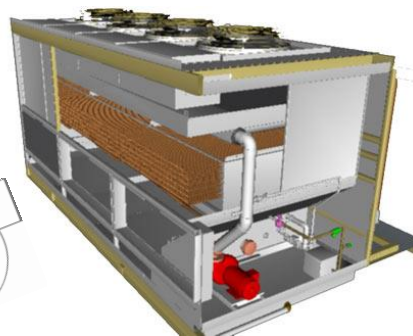
水冷式冷却器 Water-Cooled Chiller
