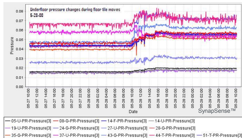
地板下面压力 under-floor pressures
