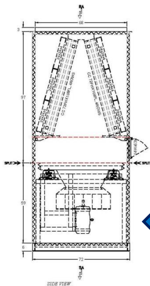
空气处理单元 CRAH
