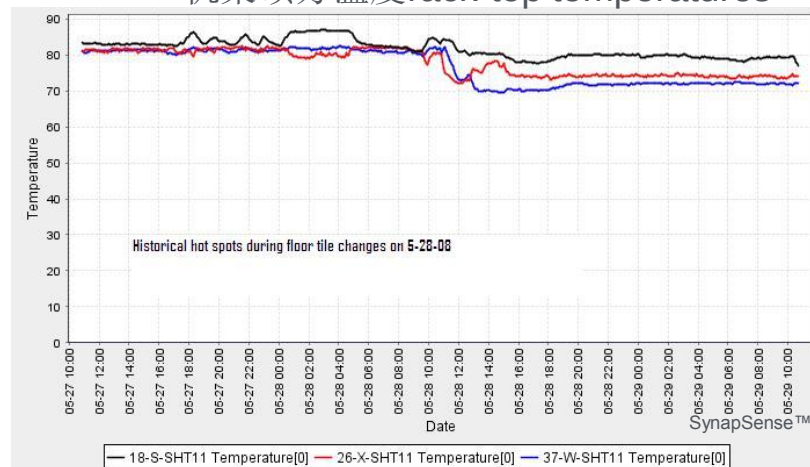
机架顶方温度 rack-top temperatures
